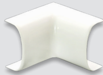
Inneneck Art-Nr.1045 Winkel: 90 ° Werkstoffgüte: PC-ABS Halogenfrei: Ja Verpackungseinheit: 40 Stück
